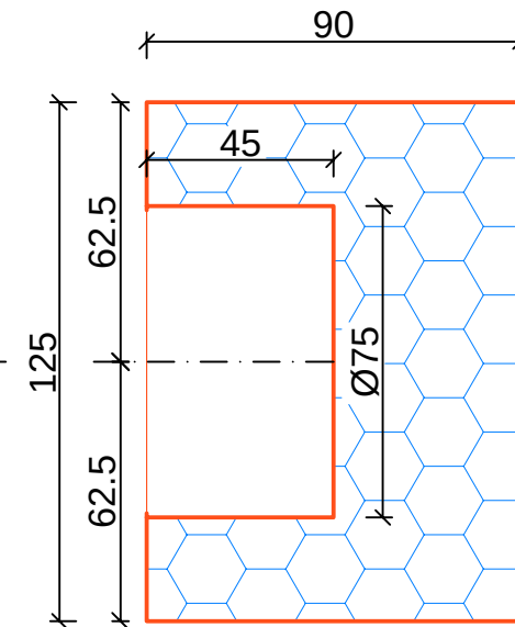
ŘEZ BLOKEM
