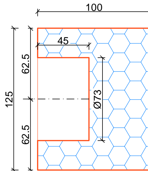
ŘEZ BLOKEM
