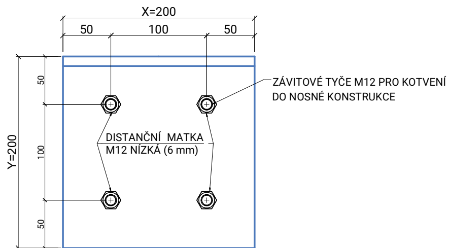
POHLED ZADNÍ
