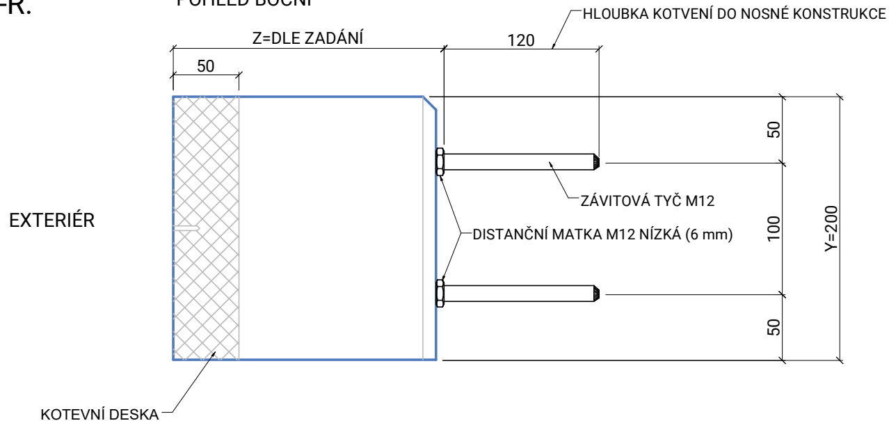
POHLED BOČNÍ
