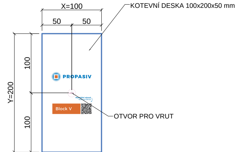
POHLED PŘEDNÍ
