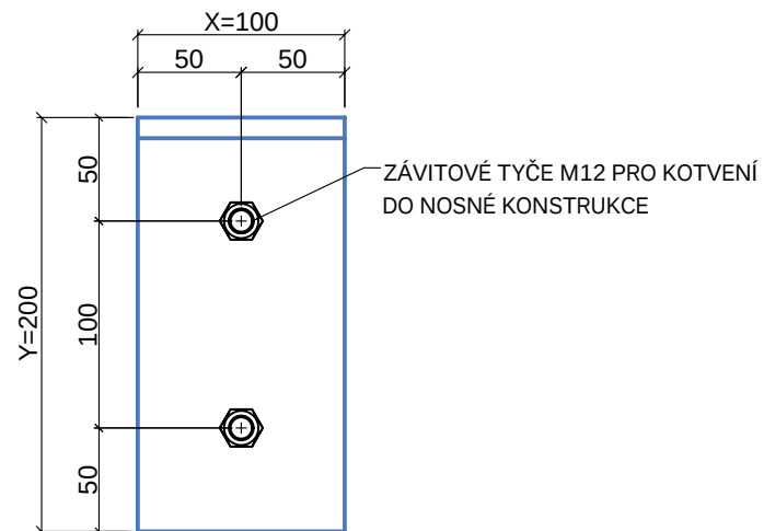
POHLED ZADNÍ
