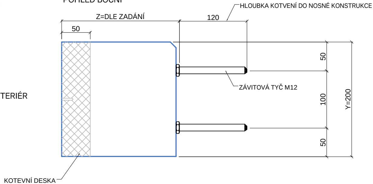
POHLED BOČNÍ
