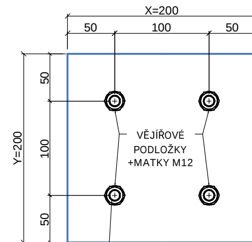
POHLED PŘEDNÍ
