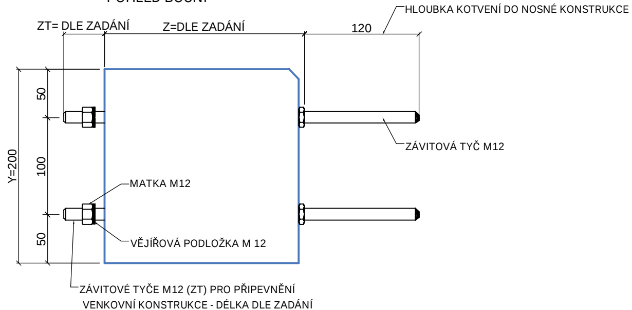
POHLED BOČNÍ
