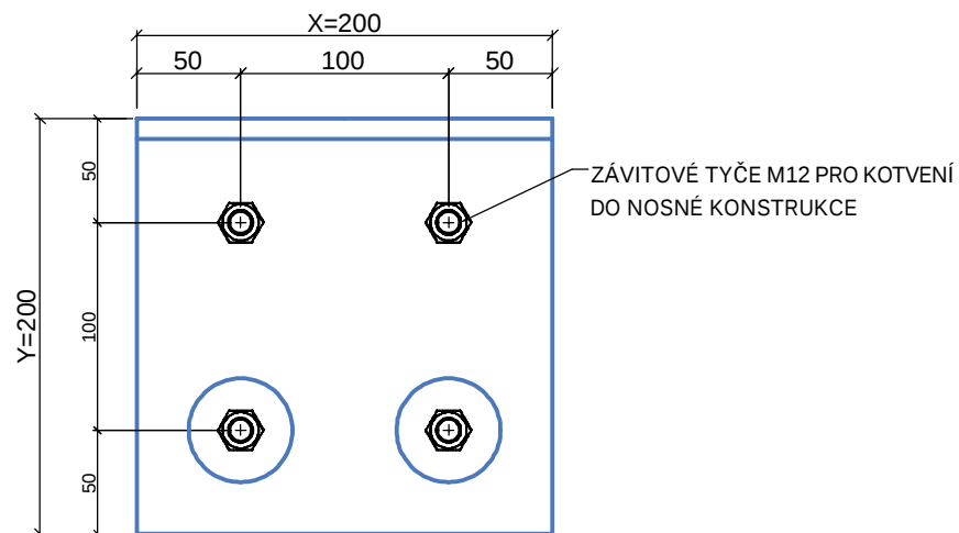
POHLED ZADNÍ
