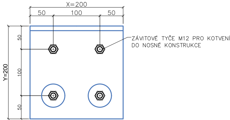
POHLED ZADNÍ
