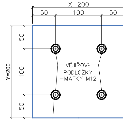
POHLED PŘEDNÍ
